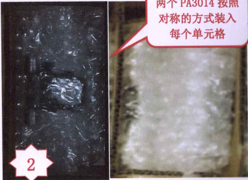
图二，用一个气泡袋包装一个 PA3014，每个单元格放入 2 个包装好的 PA3014
